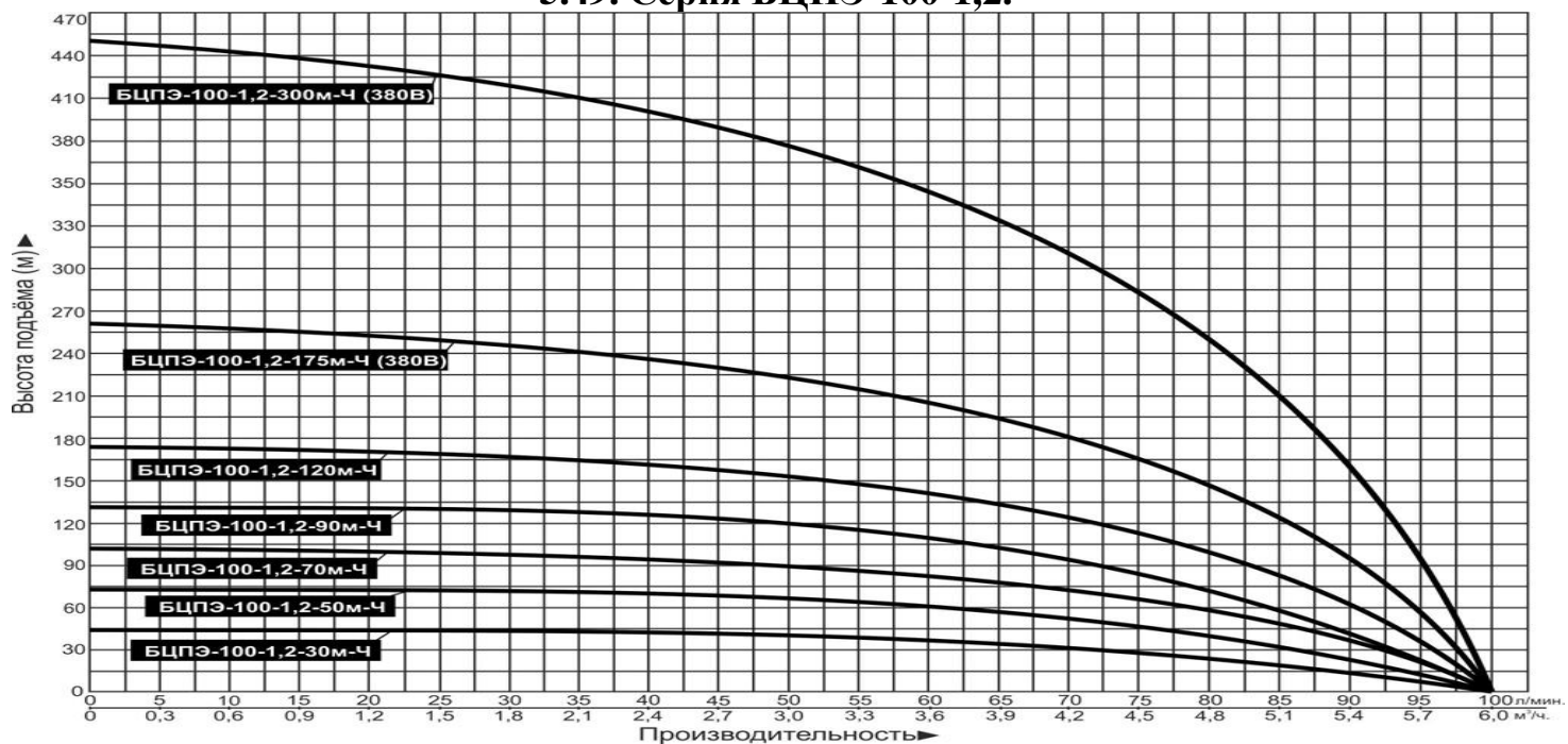
5.49. Серия БЦПЭ-100-1,2.
