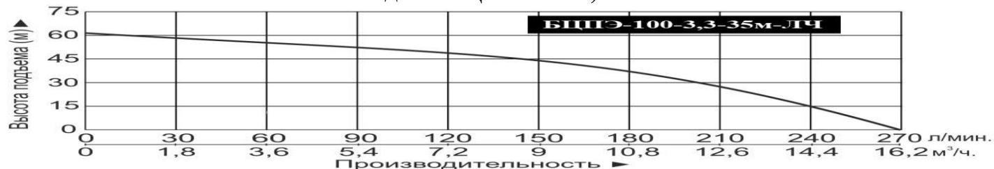
5.27. Модель БЦПЭ-100-3,3-40м-ЛЧ.
